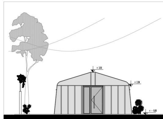
VISTA A-A
