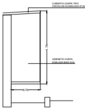
CORTE Esc. 1:25
