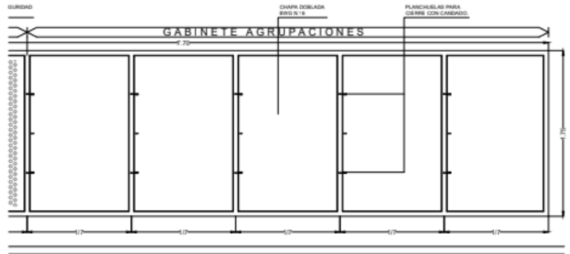
VISTA Esc. 1:25
